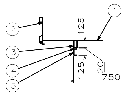
A-A SECTION
