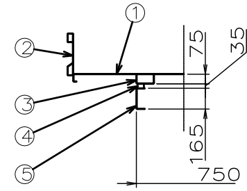
A-A SECTION
